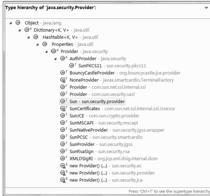
图3-3 Provider类及其子类
