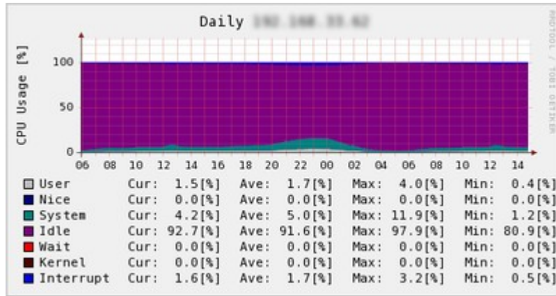
图 5.5: CPU 利用率
