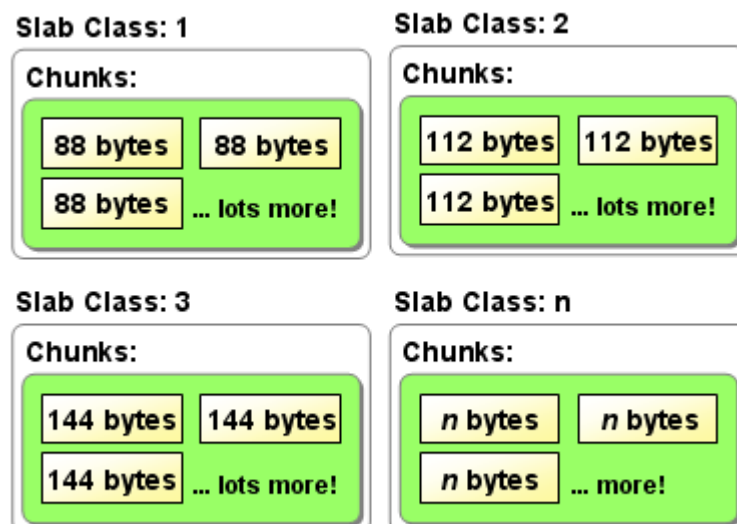
图 2.1: Slab Allocation 的构造图
