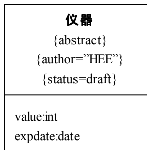
图 2.14 仪器类的性质示例
