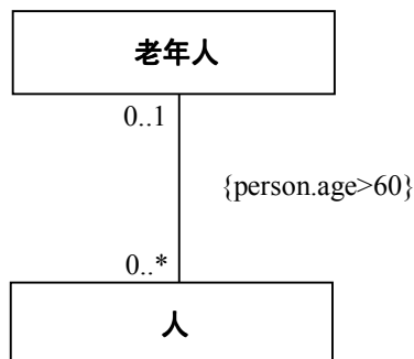
图 2.15 约束示例
