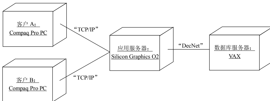
图 2.9 展开图示例
