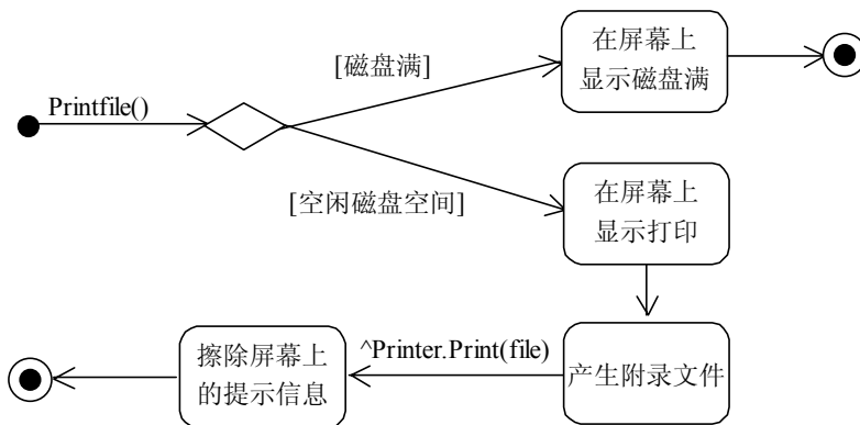
图 2.7 活动图示例
