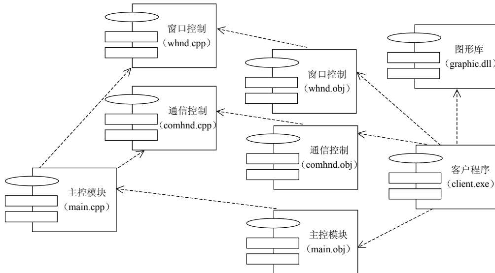
图 2.8 组件图示例
