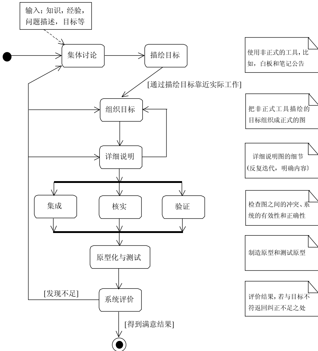
图 2.17 实际建模工作的大致流程
