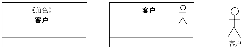
图 2-13 版类的图示方法
