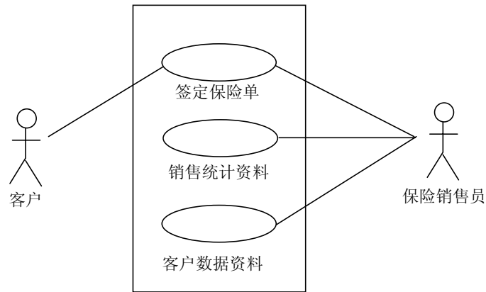
图 2.1 用例图示例
