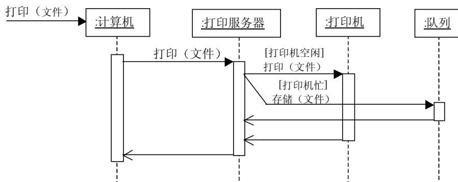
图 2.5 序列图示例
