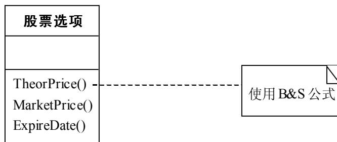
图 2.12 笔记图示
