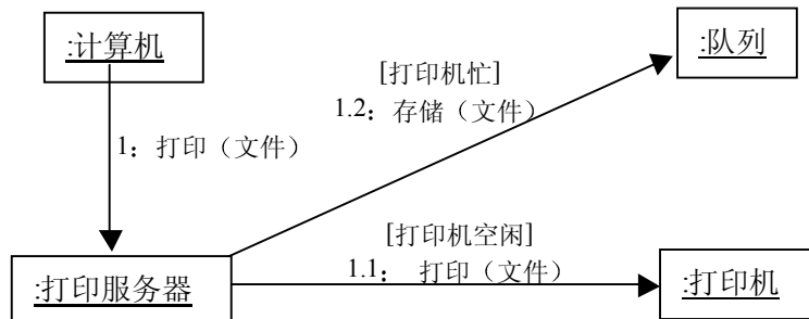
图 2.6 协作图示例
